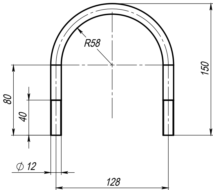
Поз.5 (Хомут)
