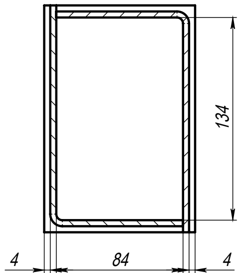
Поз.4 (Подушка)
