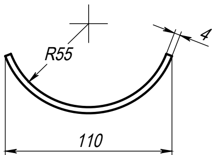
Поз.4 (Подушка)
